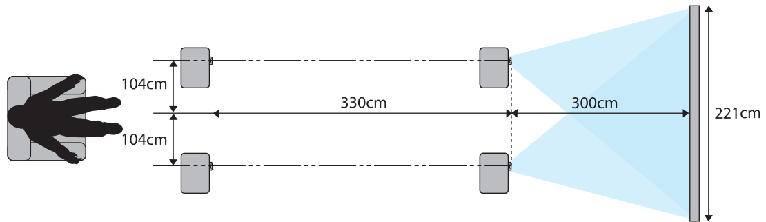
Вид сверху
