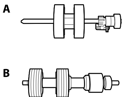
А: листоподаваща ролка, В: разделителна ролка
